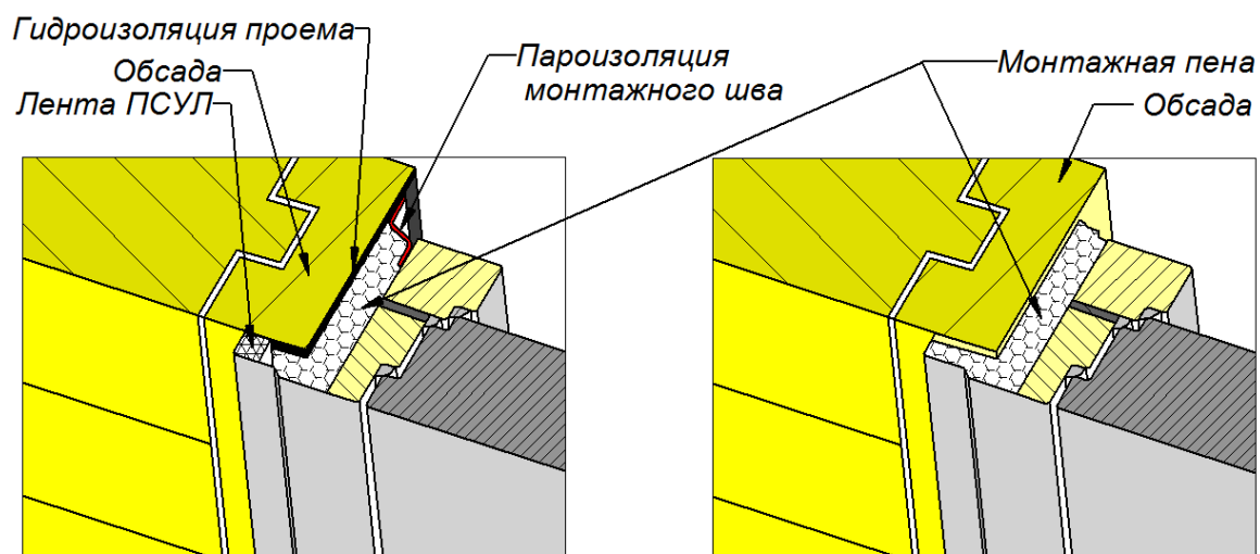
Рис. 11 Схема ПРАВИЛЬНОГО монтажа дверного блока в проеме деревянного дома (Выполнена гидроизоляция проема, наклеена лента ПСУЛ по периметру наличника, выполнена пароизоляция монтажного шва)
